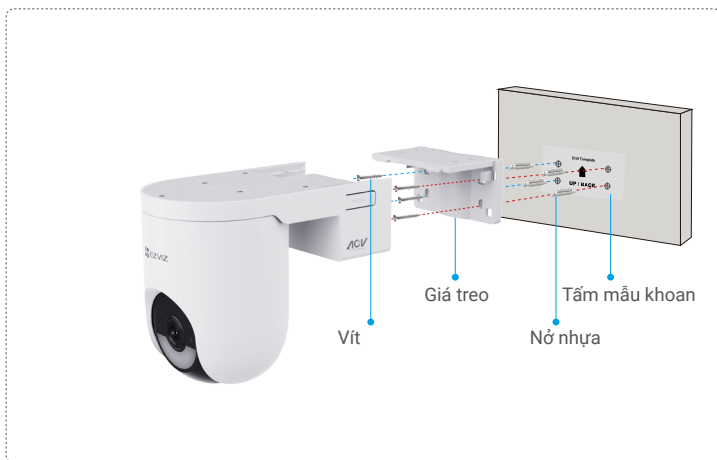
Hình 2 Gắn tường
